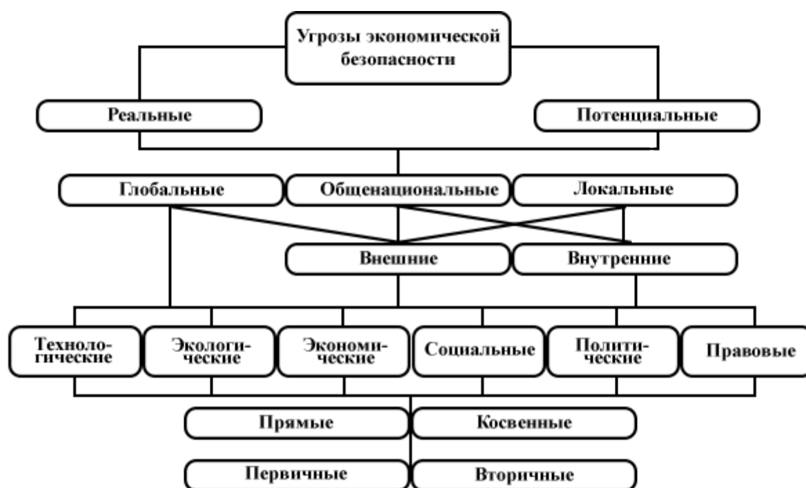
Рис. 1 – Схема угроз экономической безопасности РФ
